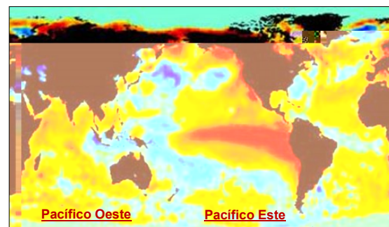
Figura 1 - Calentamiento de la TSM
