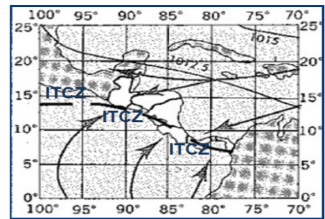
Figura 1 - ITCZ, MES DE SEPTIEMBRE
